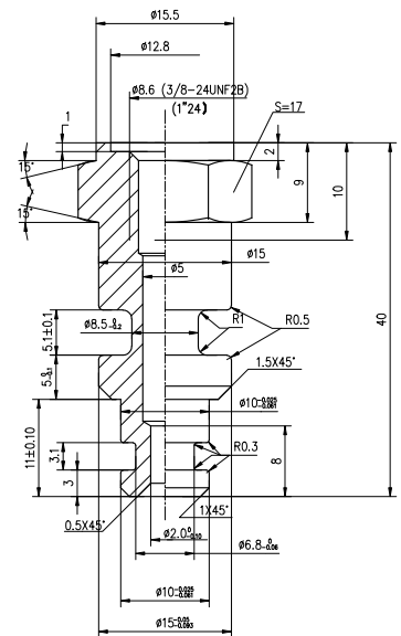
(DN6)
