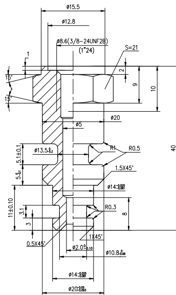
(DN10)
